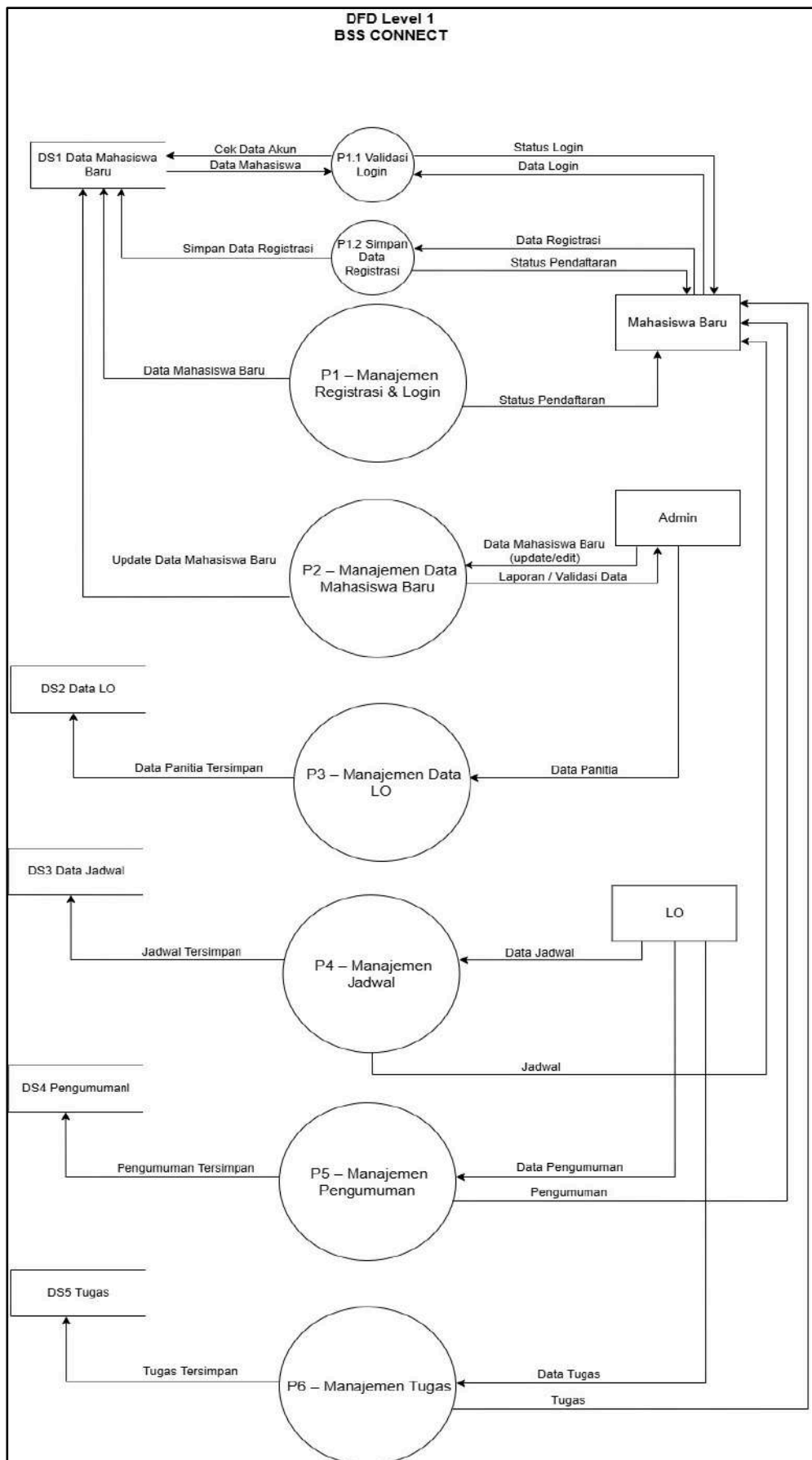
Gambar 3. 4 DFD Level 1
