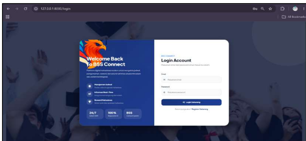
Gambar 4. 2 Halaman Login
